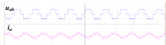
(d) Results of six-step operation
