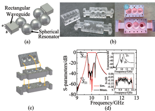
图 6 基于单模球形谐振器的 10 GHz 3-D 打印五阶带通滤波器 [57] . (a) 几何构形(矩形波导口宽高: a = 22.86 mm, b = 10.16 mm); (b) 加工的滤波器模块照片(左: 镀铜前; 右: 镀铜后; 铜层厚度 25 \mu\text{m} ); (c) 滤波器装配示意图; (d) 仿真与测量结果
