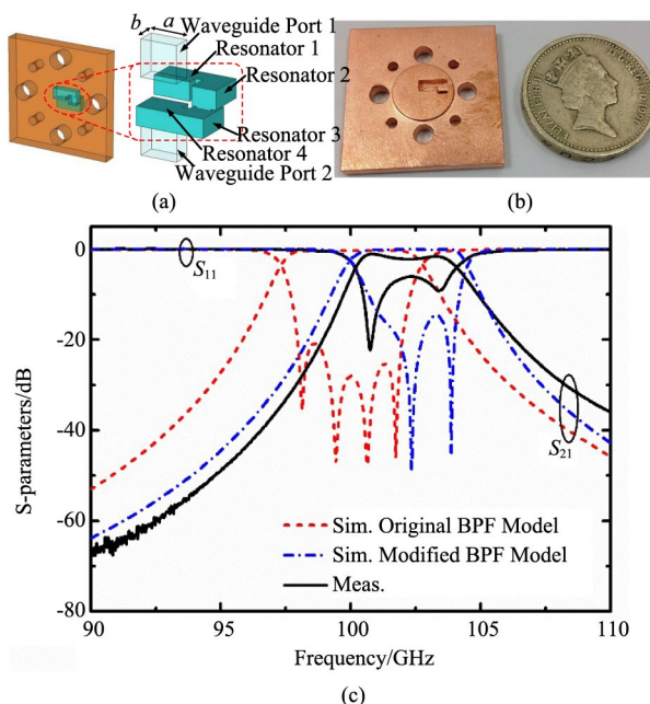
图9 100-GHz 3-D打印紧凑片上结构四阶带通滤波器. (a) 结构示意图(矩形波导口宽高: a = 2.54 mm, b = 1.27 mm);(b) 加工的滤波器照片;(c) 仿真与测量结果
