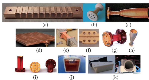
图 2 基于“非金属打印+表面金属化”模式的 3-D 打印毫米波器件 [30-37] . (a) Ka 频段宽带喇叭天线阵列 (SLA); (b) 带法兰的 WR-10 直通波导 (75~110 GHz) (SLA); (c) W 频段波纹喇叭天线 (SLA); (d) X 频段波导缝隙天线阵列 (SLA); (e) WR-90 直通波导 (8.2~12.4 GHz) (FDM); (f) W 频段六阶波导带通滤波器 (SLA); (g) WR-3.4 直通波导 (220~330 GHz) (SLA); (h) 92.5-GHz 波纹喇叭天线 (SLA); (i) WR-3.4 频段对角线喇叭天线 (SLA); (j) 内表面金属化的直通波导 (FDM); (k) Ku 频段波纹圆锥喇叭天线 (FDM)
