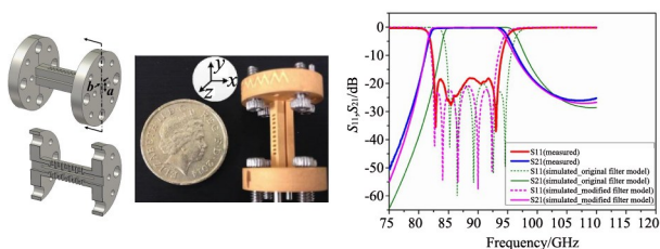
图8 90-GHz 3-D打印裂缝波导五阶带通滤波器 [67] . (a) 结构示意图(矩形波导口宽高: a = 2.54 mm, b = 1.27 mm);(b) 加工的滤波器照片;(c) 仿真与测量结果
