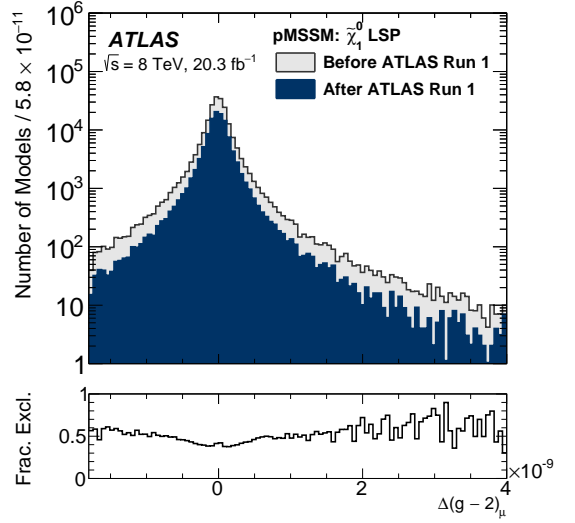
(d) Muon magnetic moment
